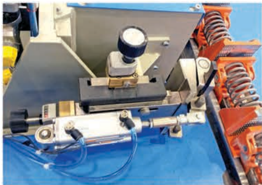
KONTIZINK glue applicator with matrix. KONTIZINK Leimauftrag mit Kamm.
