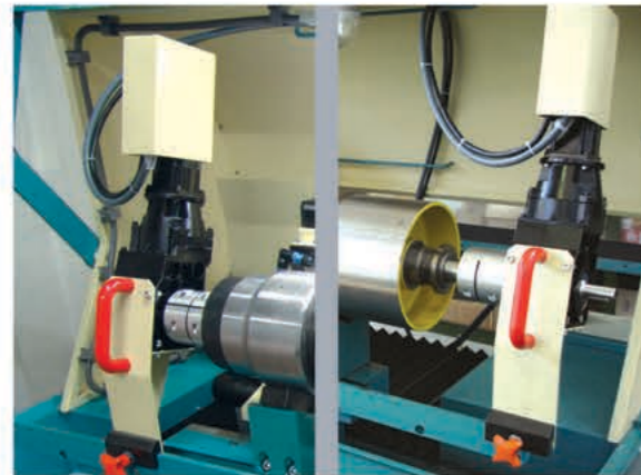
Servo indexing unit, attachable left/right. Servoteilapparat links/rechts aufsetzbar.
