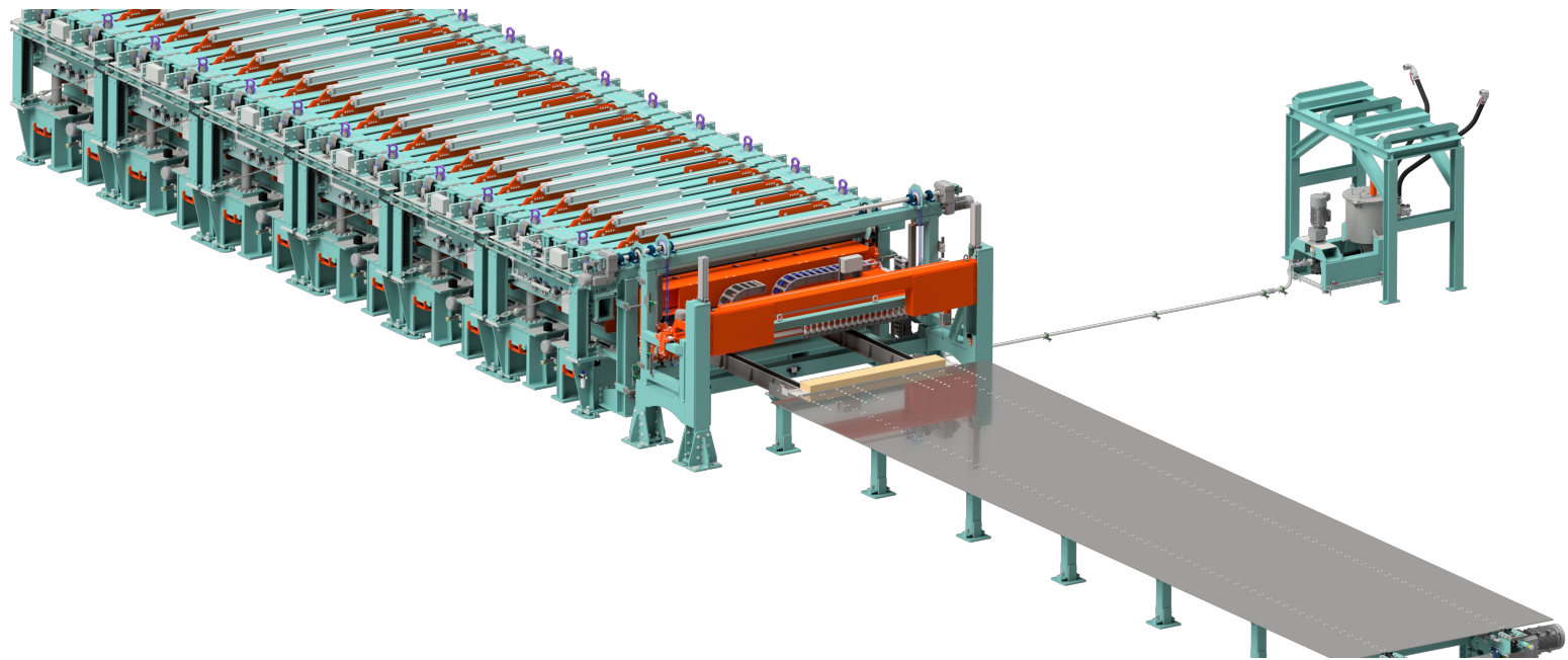
LEDINEK DE - LEIMHOLZANLAGEN - XE-PRESS
