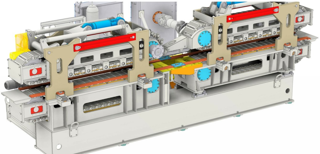
LEDINEK DE - KEILZINKEN - KONTIZINK H 3000
