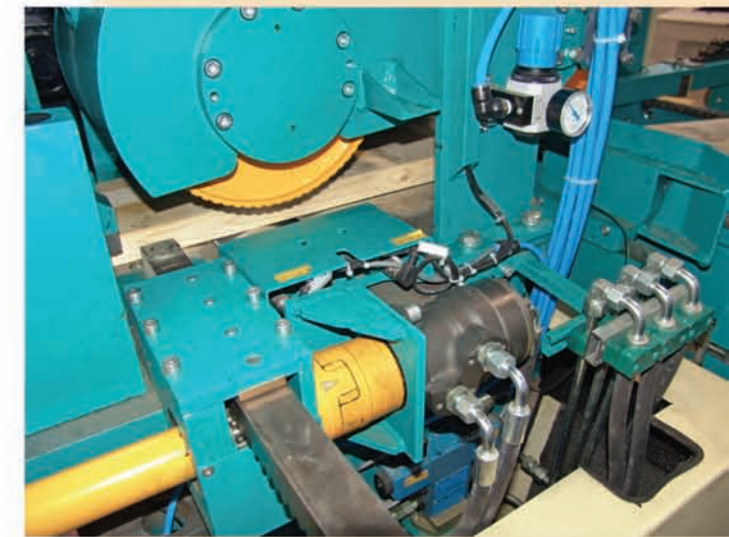
Starke hydraulische Lineale richten das Brett seitlich aus. Powerful hydraulic side fences align and straighten the board.
