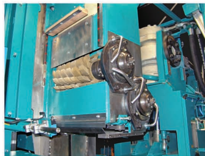
Doppelte Fräseinheit mit Hochleistungsspindeln und Gegenlagern. Double milling unit with heavy-duty spindles and support bearings.
