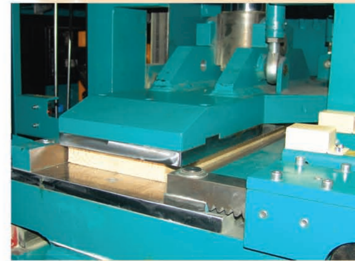
Bretter werden von oben geklemmt; einkommendes Brett wird auf die Lamelle verpresst. Boards are clamped from top; inbound board is pressed to the lamination.
